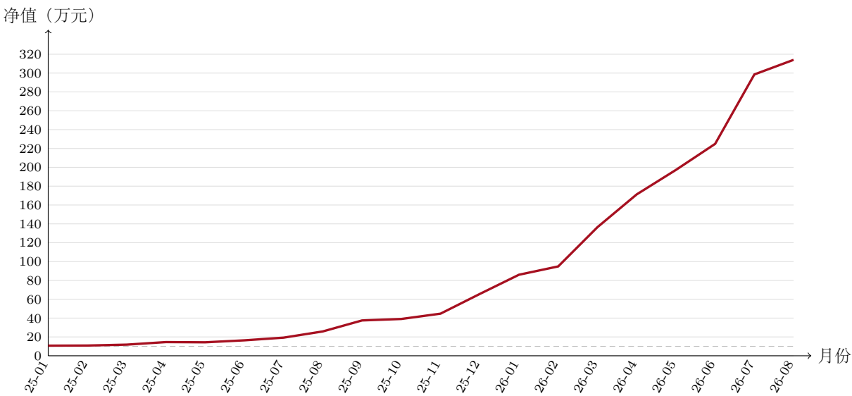
图 1: 信号日复利净值（本金 10 万元）。虚线为起始本金。
